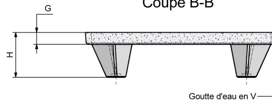
ELEMENT SUPERIEUR Coupe B-B
