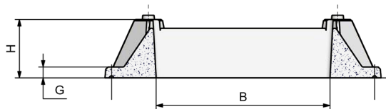
ELEMENT DE BASE Coupe A-A
