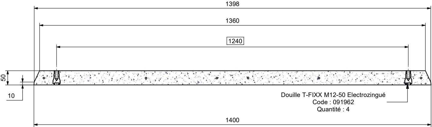
A-A ( 1 : 8 )
