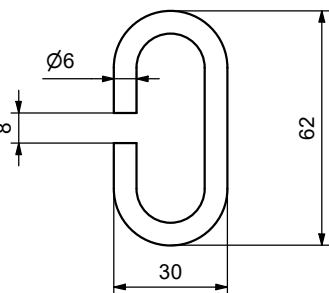
Détail d'un anneau pour fixation chaîne (Quantité : 2)
