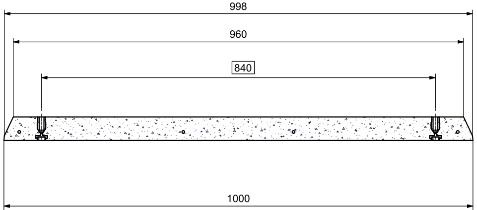
B-B ( 1 : 8 )
