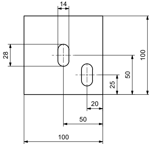
Détail d'une platine Ep.5 mm (Quantité : 4)
