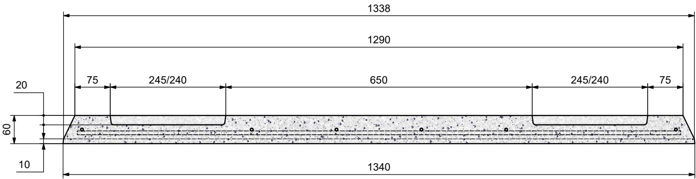
A-A ( 1 : 8 )
