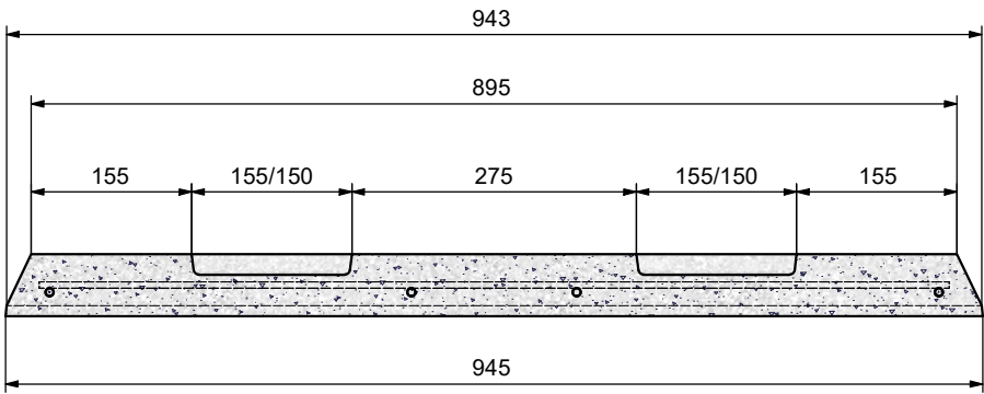
B-B ( 1 : 8 )
