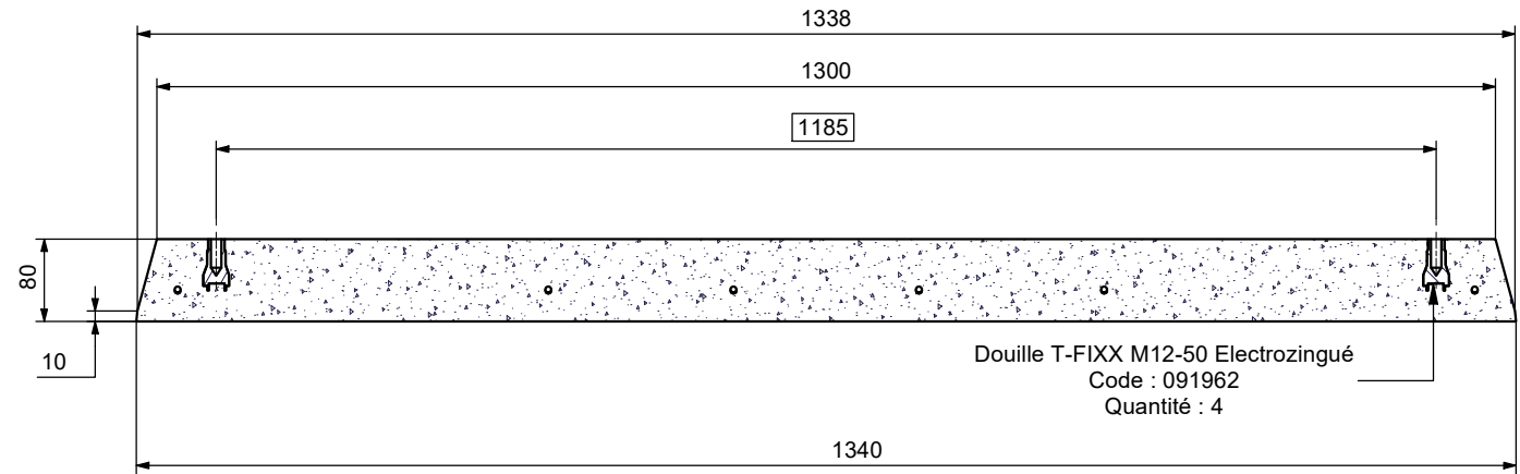
A-A ( 1 : 8 )
