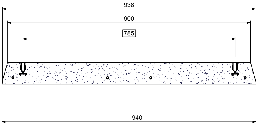
B-B ( 1 : 8 )
