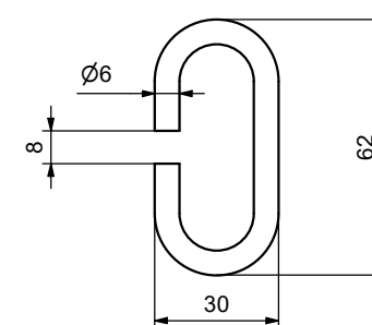
Détail d'un anneau pour fixation chaîne (Quantité : 2)
