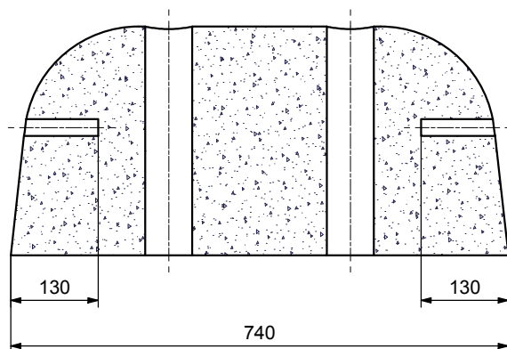
A-A ( 1 : 10 )
