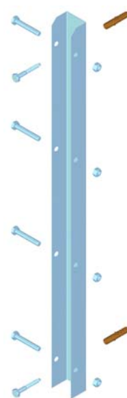
U INOX ou PVC contre Mur
